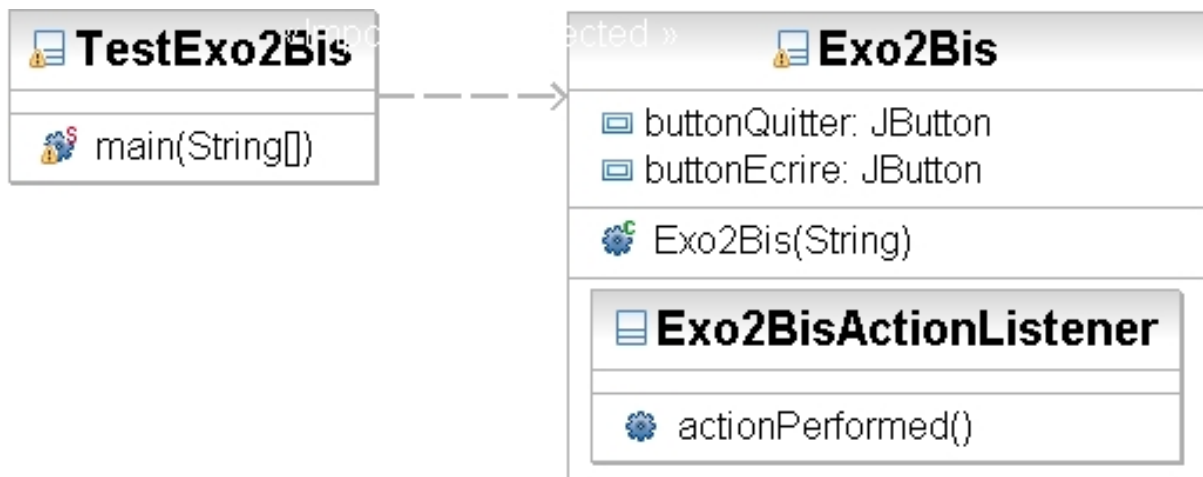
Figure 2.25. ne action sur deux boutons avec une classe interne
