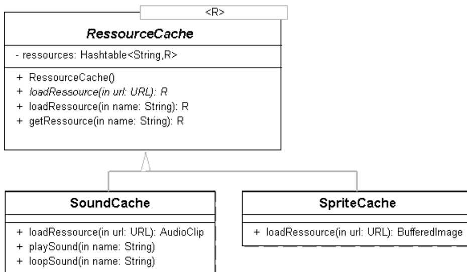
Figure 2.29. Gestionnaire de ressources
