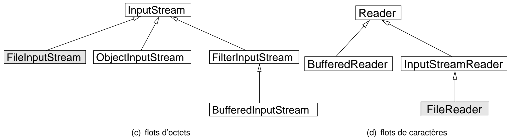
FIG. 5 – Lecture (simplifié)
