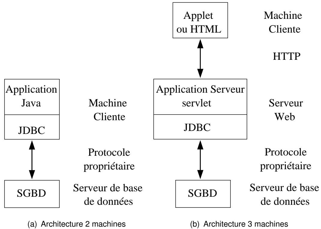
FIG. 15 – Utilisation de JDBC
