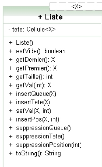
Figure 1.18. Diagramme UML de la classe Liste
