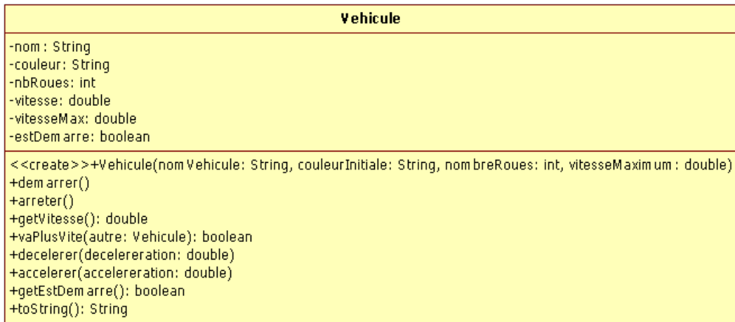
Figure 2.2. Classe véhicule
